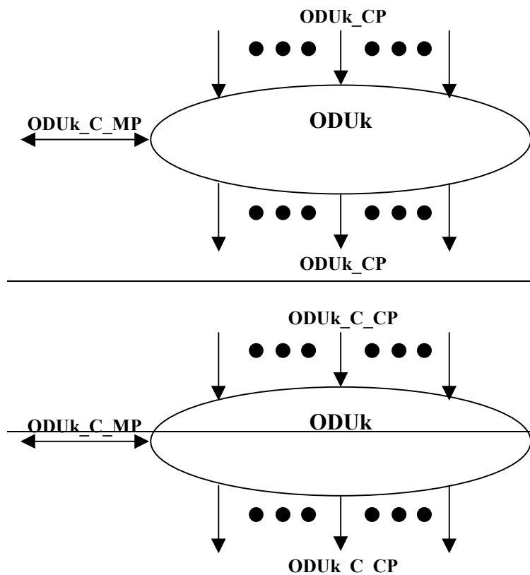
Figure 0-4/G.798 – ODUk_C function
