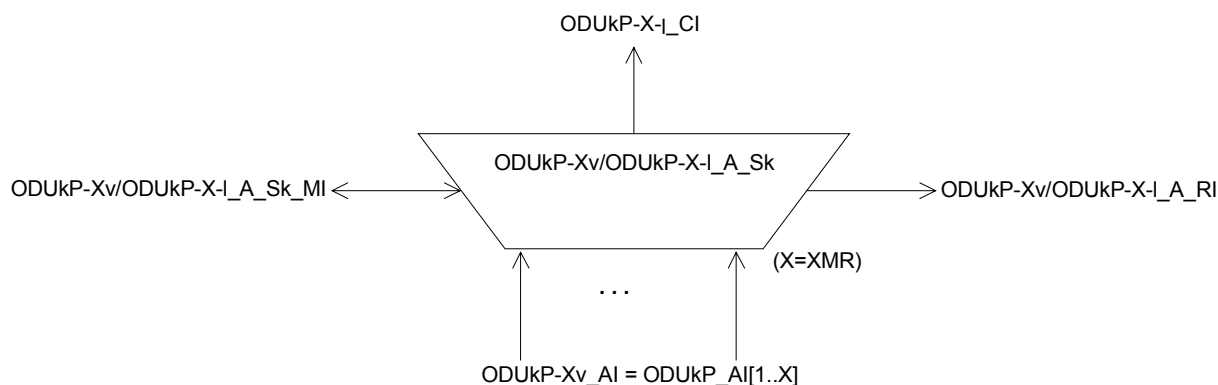
Figure 0-83/G.798 – ODUkP-Xv/ODUkP-X-L A Sk symbol
