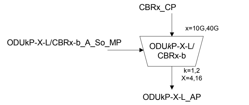
Figure 0-88/G.798 – ODUkP-X-L/CBRx-b_A_So function
